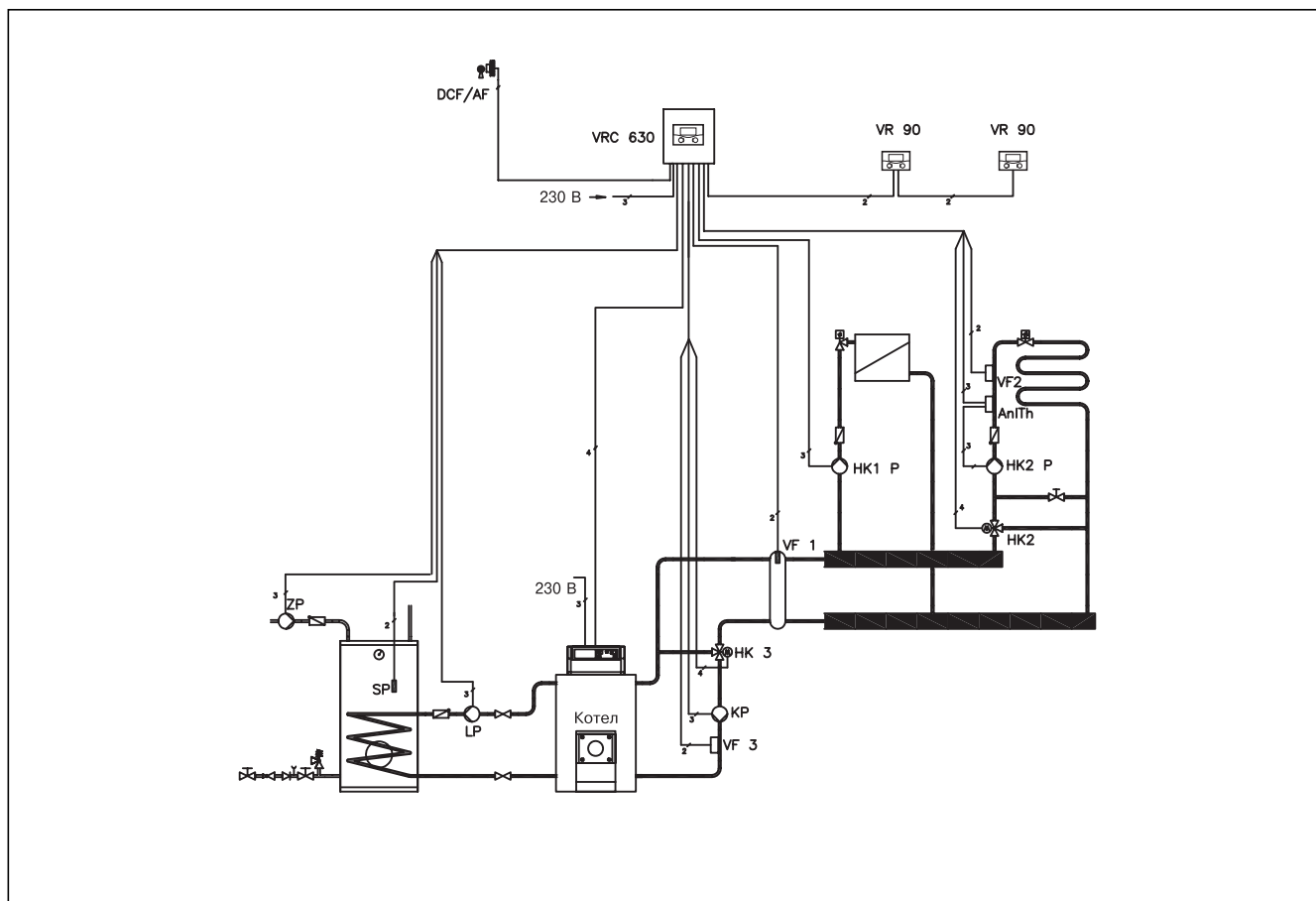
Рис. 4.12 VRC 630, подъем отводящей линии
