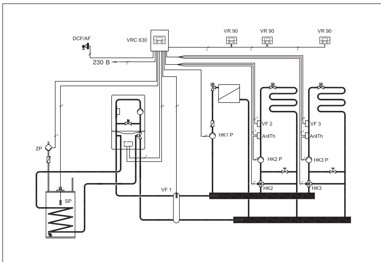
Рис. 4.4 Настенный отопительный прибор с VRC 630
