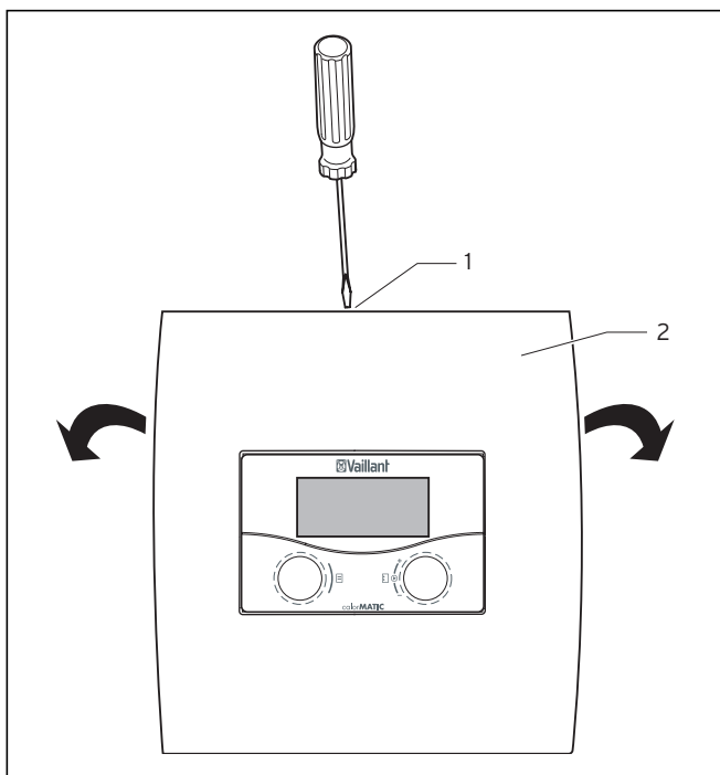
Рис. 3.2 Открытие настенной конструкции
