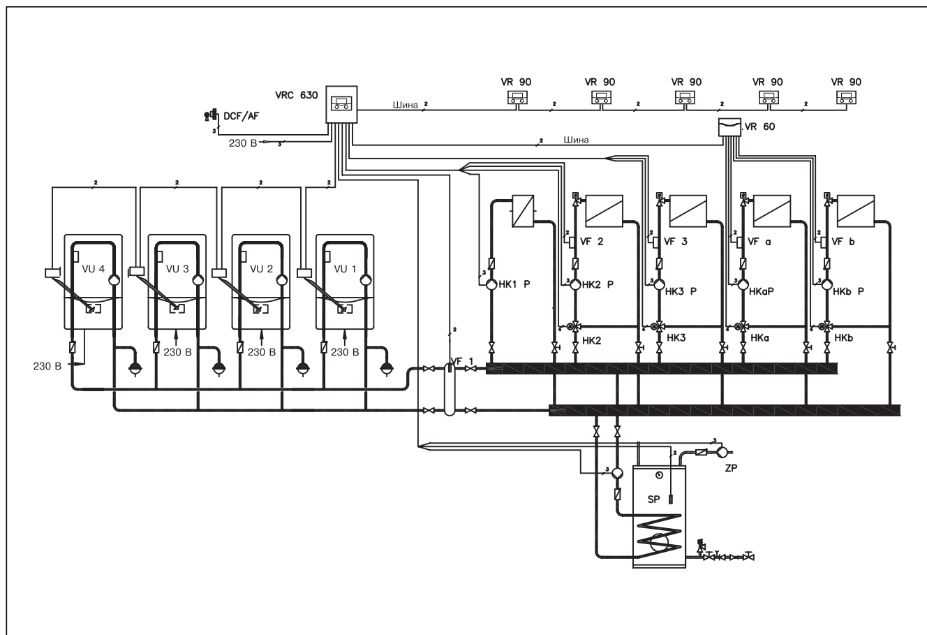
Рис. 4.8 calorMATIC 630 с 5 отопительными контурами и 4 VC 466
