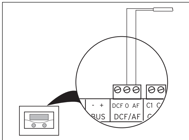
Рис. 4.16 Подключение VRC 693
